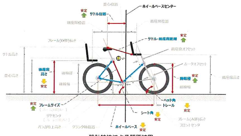
設計特性による評価結果 ※各特性の矢印の方向(増加又は減少)が走行安定性を向上させる方向を示す。
